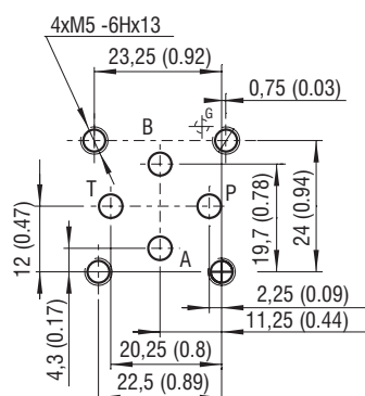
ISO 4401-02-01-0-05
