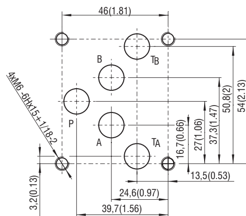
ISO 4401-05-04-0-05
