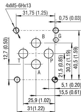
ISO 4401-03-02-0-05
