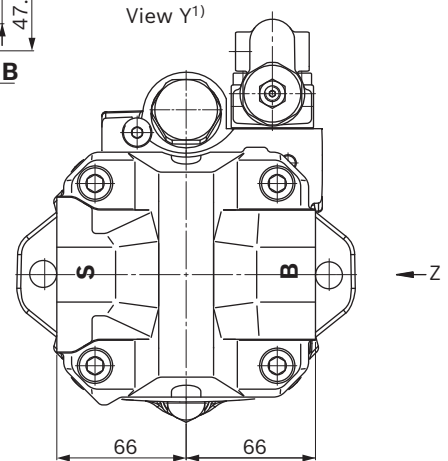
View Y 1)
