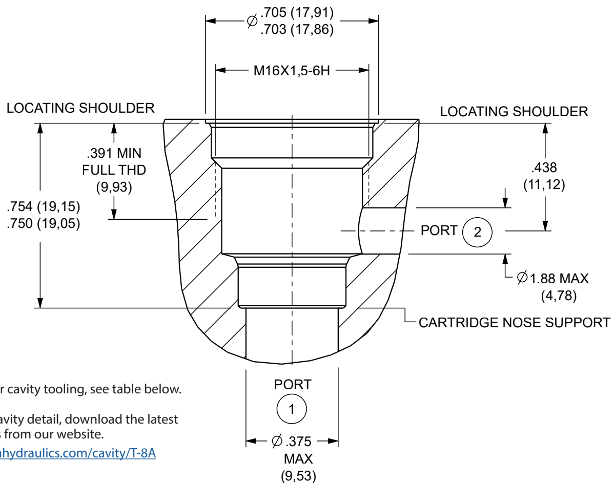
T-8A CAVITY
