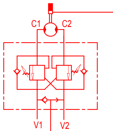
Schema Idraulico (con sbloccafreno) Hydraulic Diagram (with brake unclaping)
